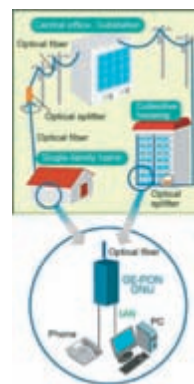
GE-PON ONU
